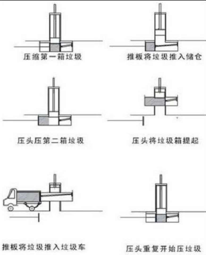
图 5-3 垂直压缩式垃圾转运操作示意图
