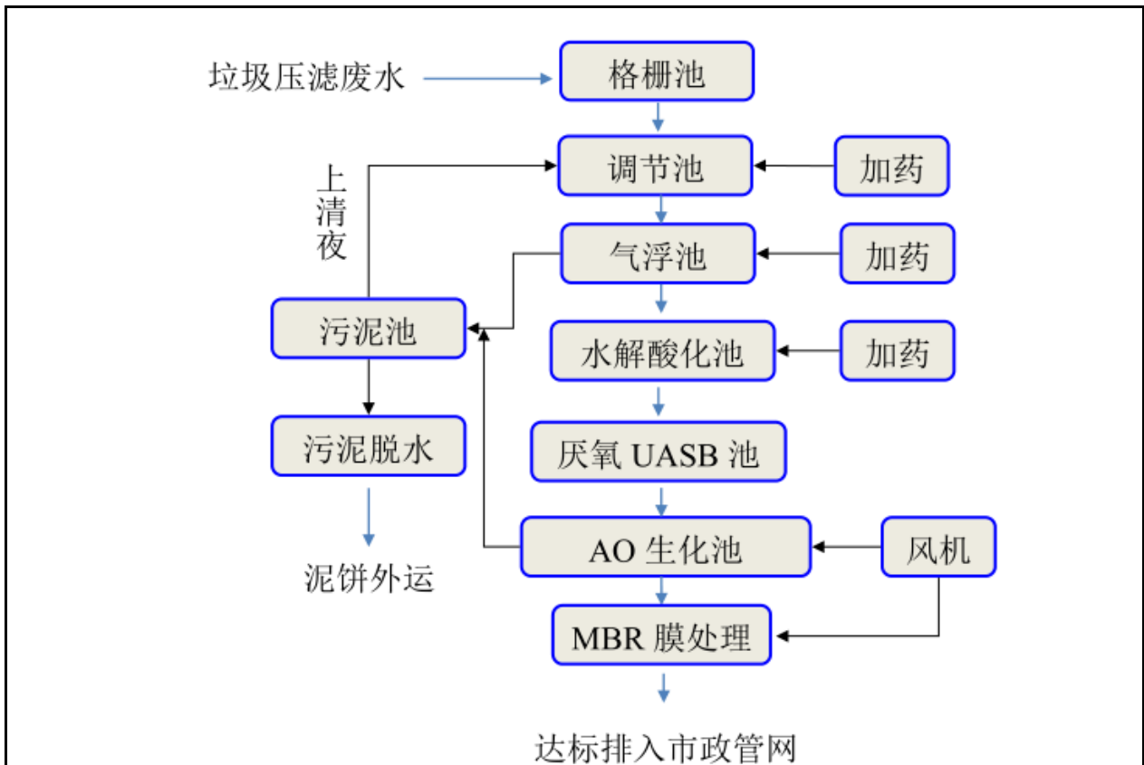
图 5-7 污水处理工艺
