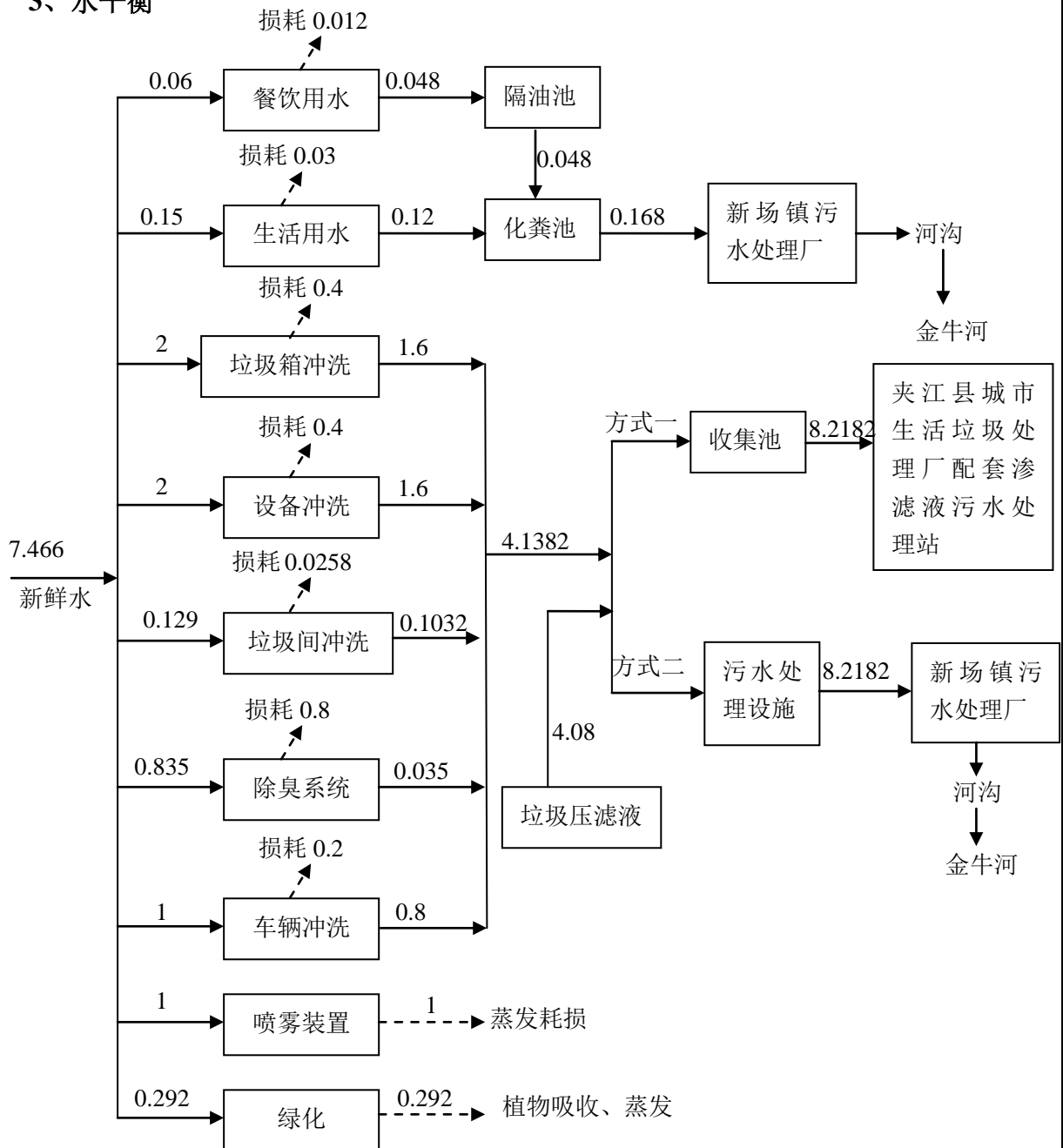
图 1-2 水平衡图
